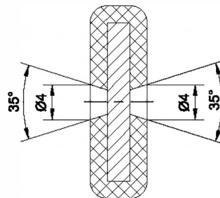
A-A (2:1)
