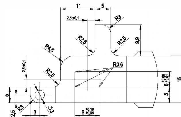
详图 A (2:1)
