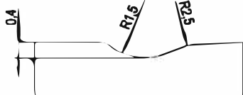
详图 B (10:1)
