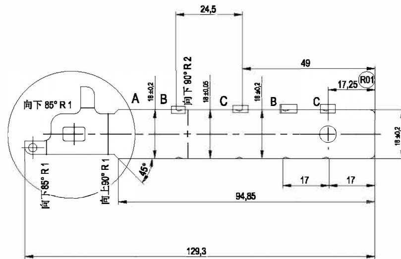
详图 A (2:1)
